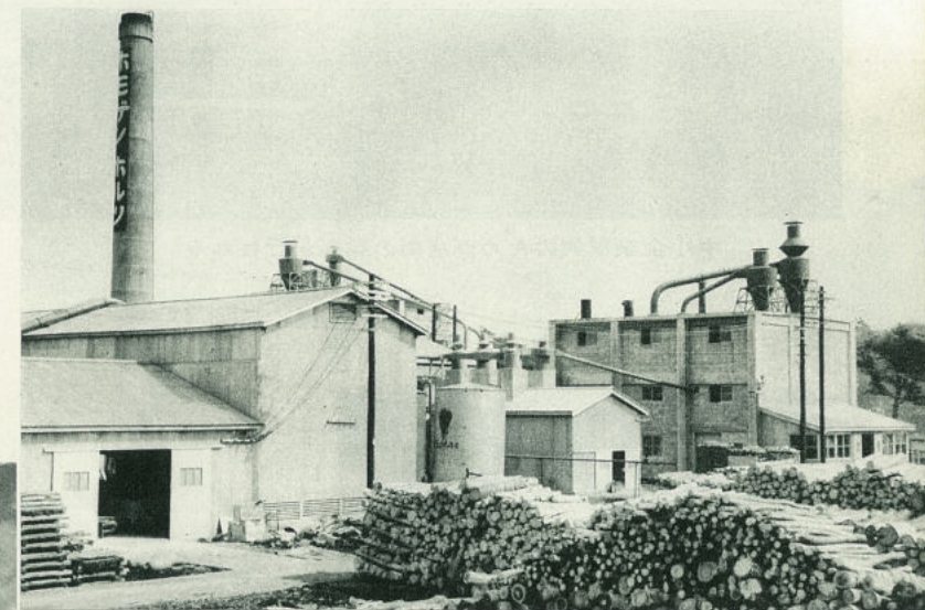
パーティクルボードを年産5千トン上げる 東北ホモボード工場
