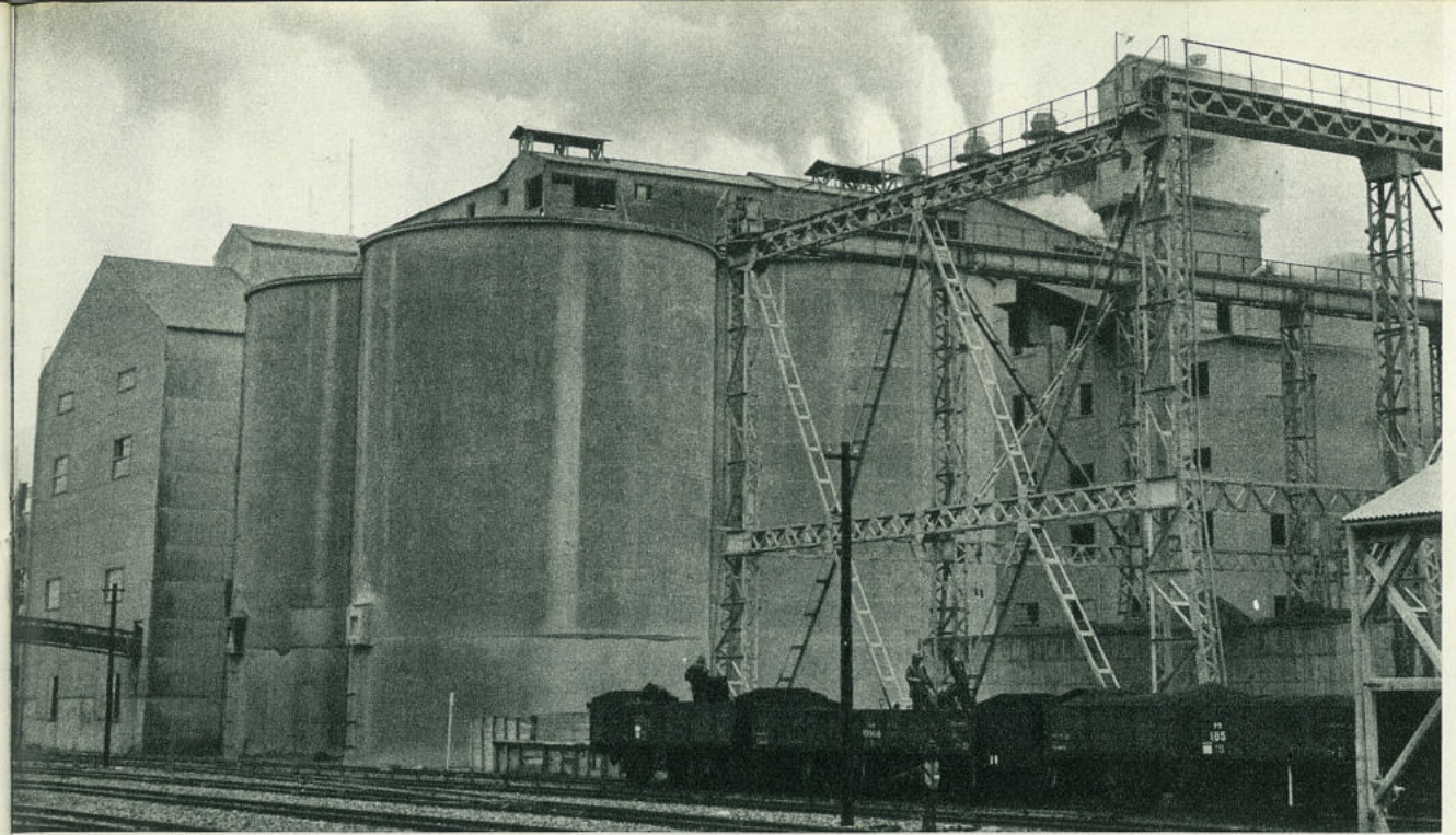
工場誘致の花形岩手セメント工場、ポルトランドセメント年産22万トン
